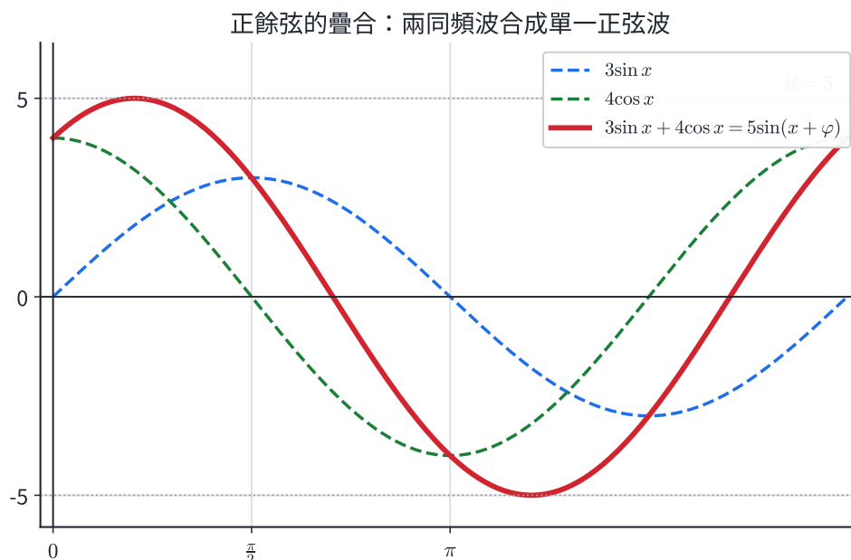
圖 1-5：兩個同頻的 \sin 與 \cos 相加，合成後仍是同頻率的正弦波，振幅變為 R = \sqrt{a^2 + b^2} 、相位移為 \varphi 。
